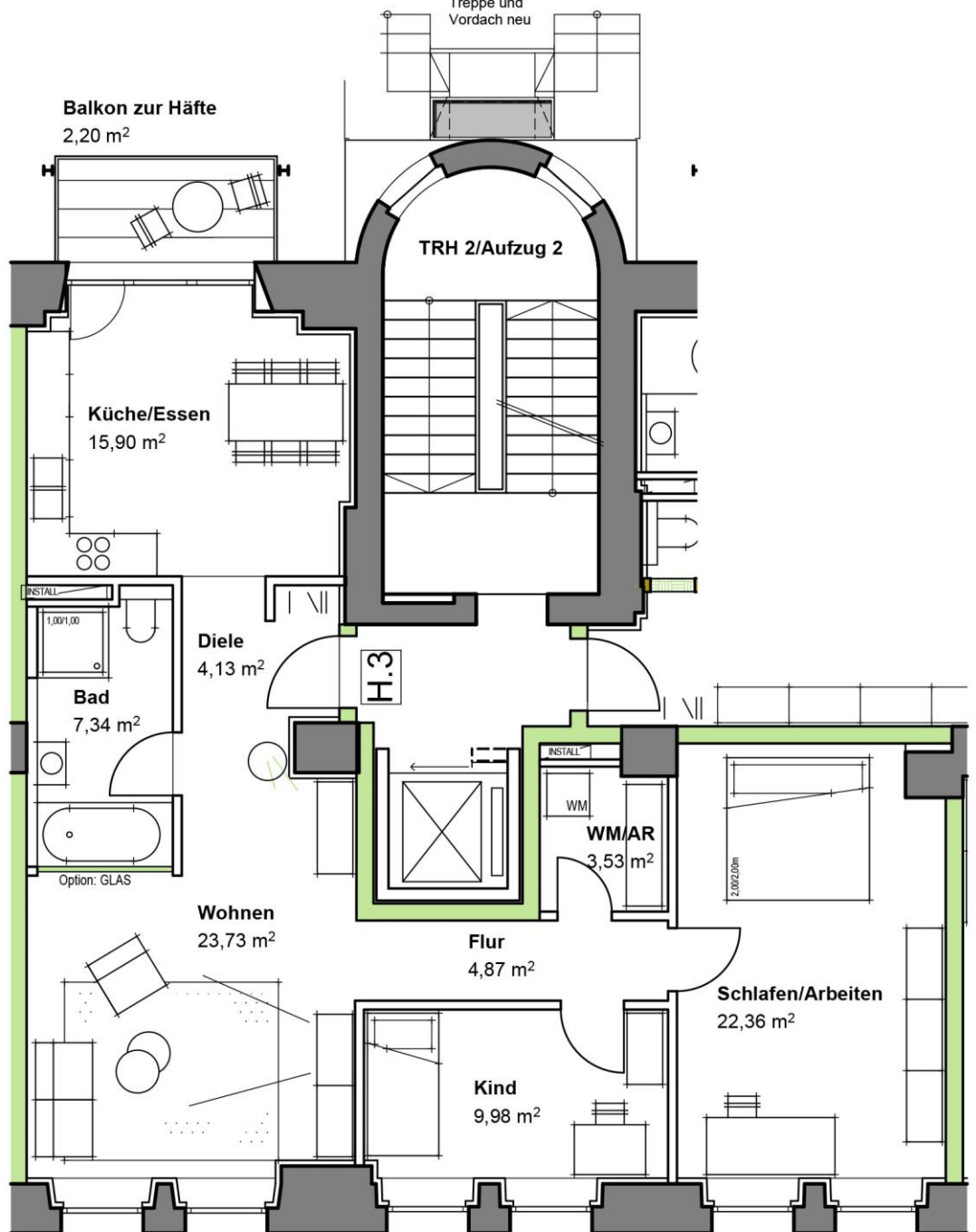
H.3: 3-Zimmer + Wohnküche
